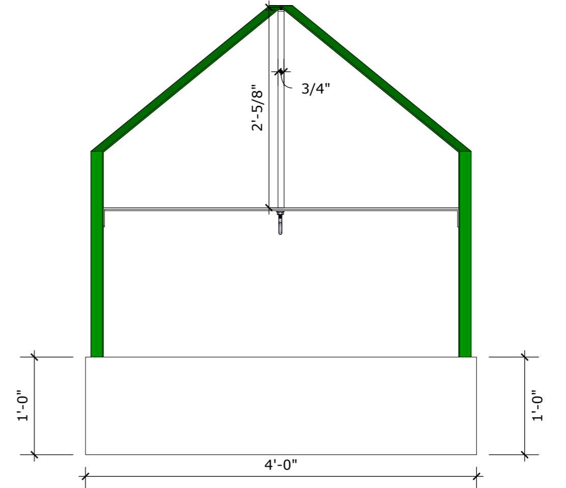
ELEVATION
